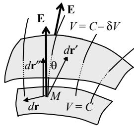
Figure 2.2. Equipotential surfaces
